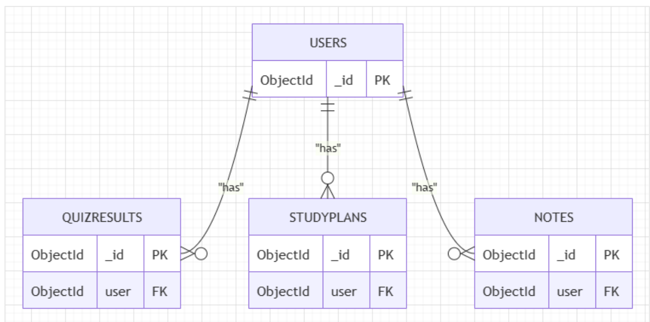
Figure : ER Diagram
